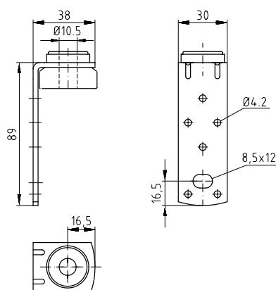
Úhelník vzduchovodu Typ I
