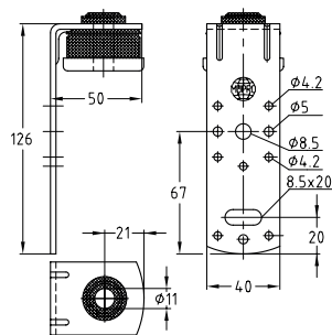
Úhelník vzduchovodu typ II
