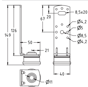
Úhelník vzduchovodu typ III
