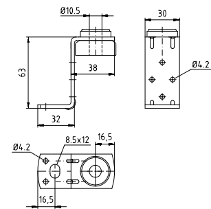
Dvojitý úhelník vzduchovodu typ I
