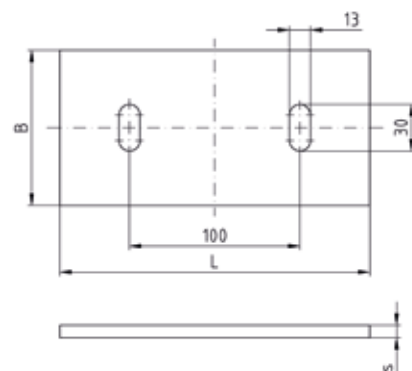
Pro profily Q50, Q100, Q150 (délka 200 mm)
