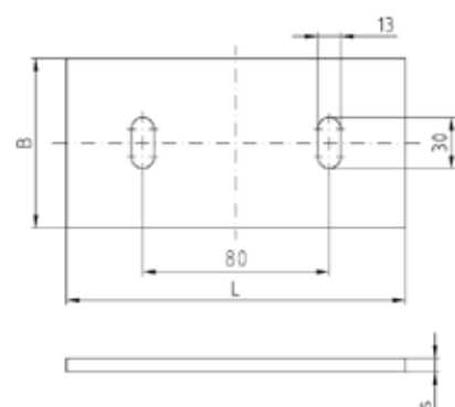
Pro profil Q80
