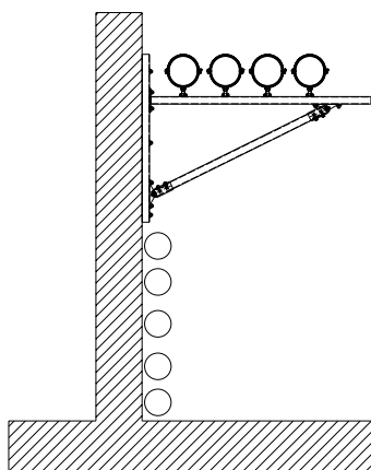
Instalace potrubí na konzole s tlačnou vzpěrou
