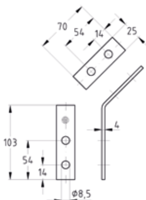
Montážní úhelník 45°
