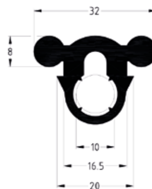
Pro nosníky 38/24 až 40/120
